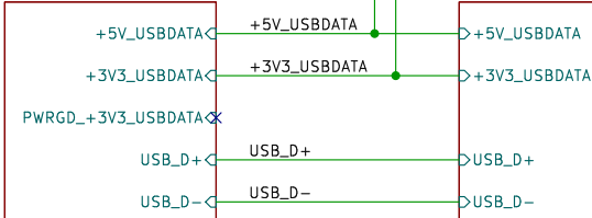
USB C #2 - Data Input
